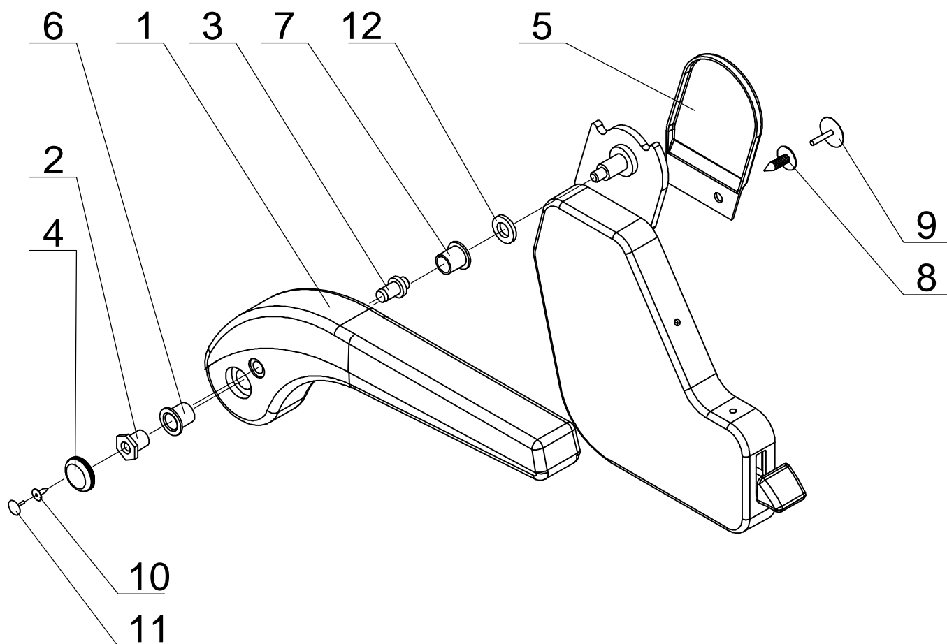
Рисунок 7 – MH15-6844010 Установка подлокотника правого MH15-6846011 Установка подлокотника левого
